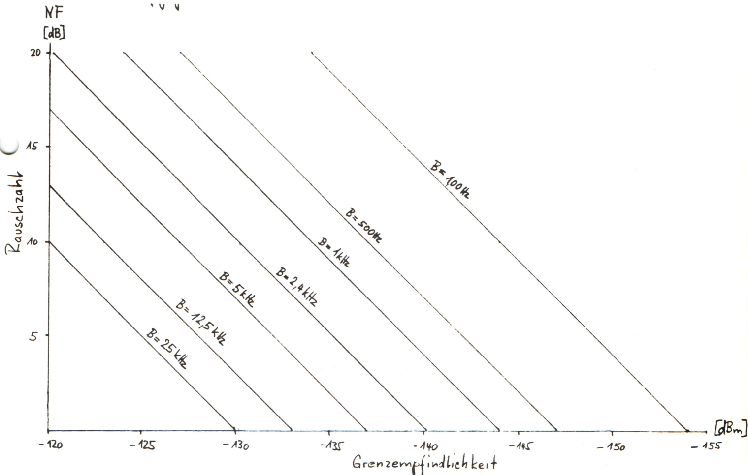
Zusammenhang von Grenzeempfindlichkeit und Rauschzahl
