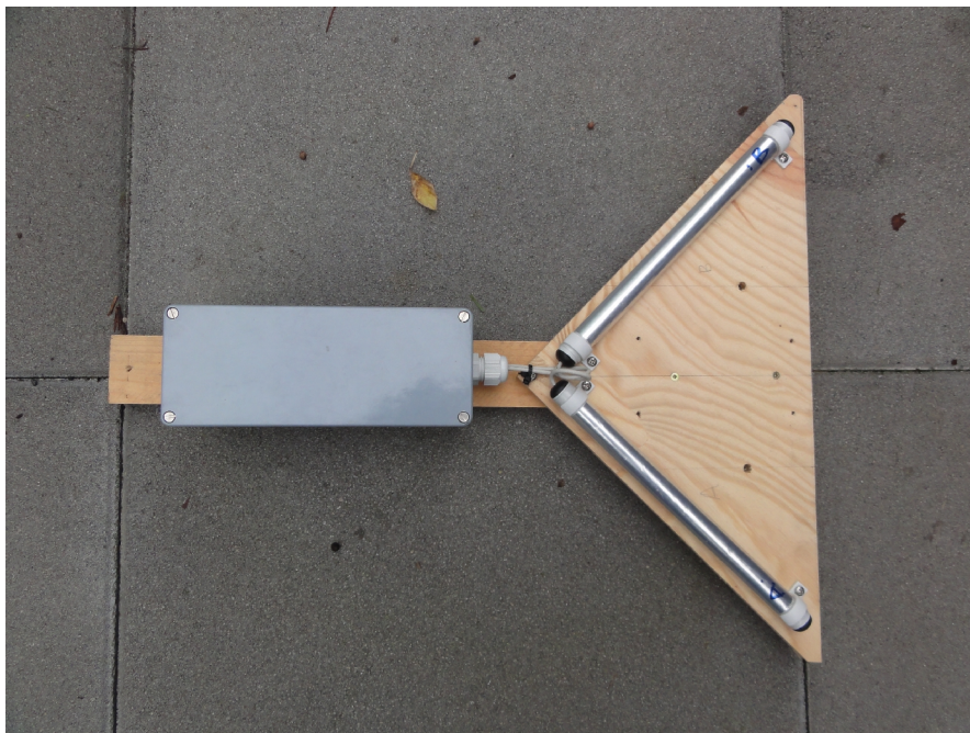
Aufbau der Empfänger
